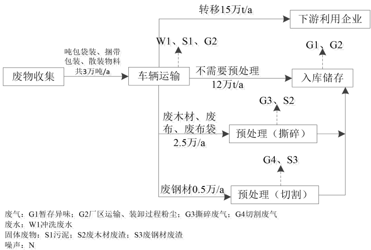
图2-2 本项目生产工艺流程及产排污节点
