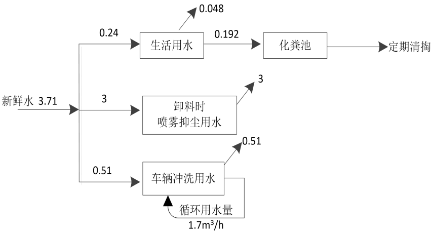
图 2-1 本项目给水排水平衡图（日最大值，单位：m³/d）
